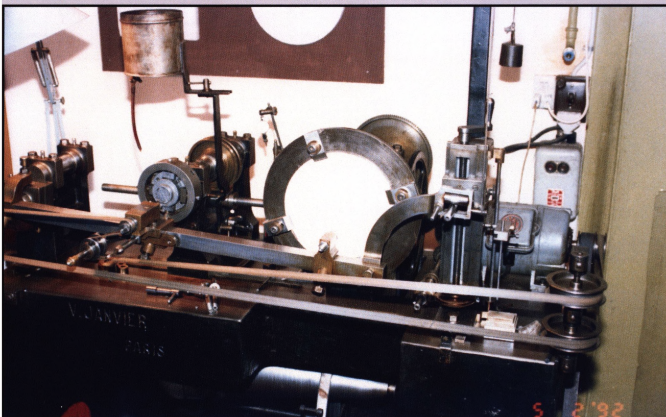
Reduktionsmaskine, hvor modellen i gips spændes op, og overføres til stålstempel. Den kgl. Mønt havde en søstermodel stående.
